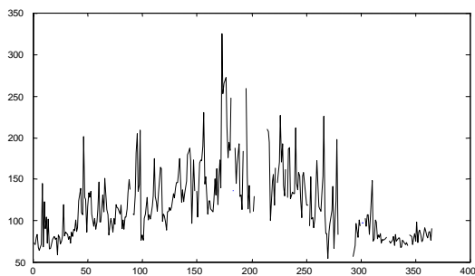
Figure 3a. Melilli, O 3 , Max per Day, 1998
